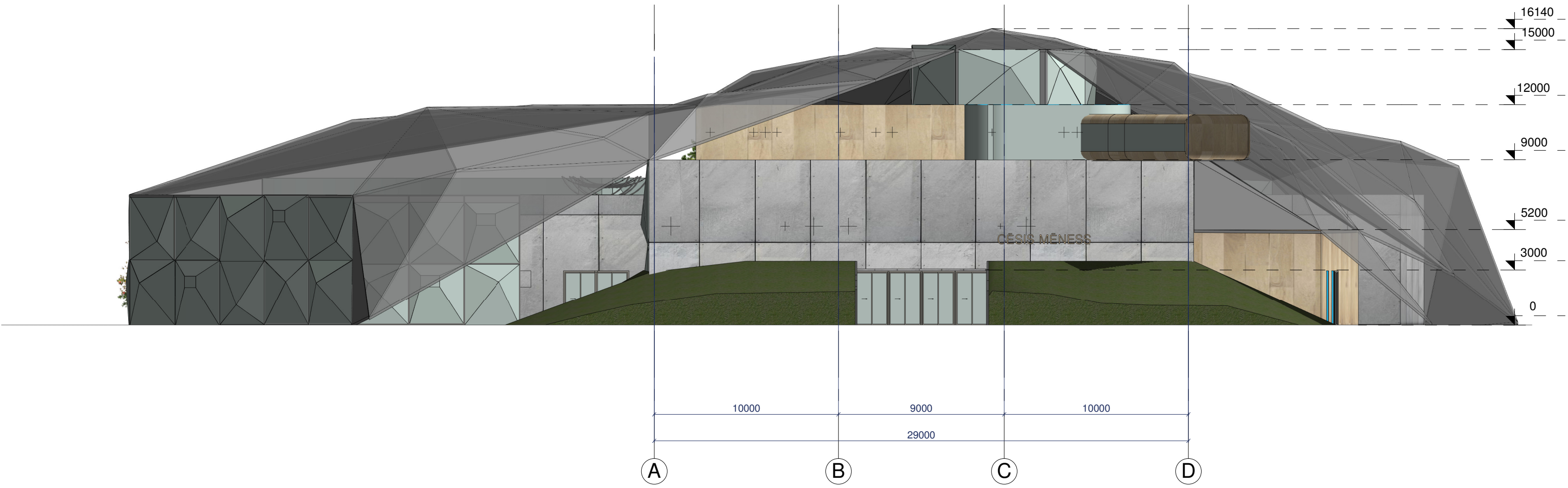
Ziemeļu fasāde
