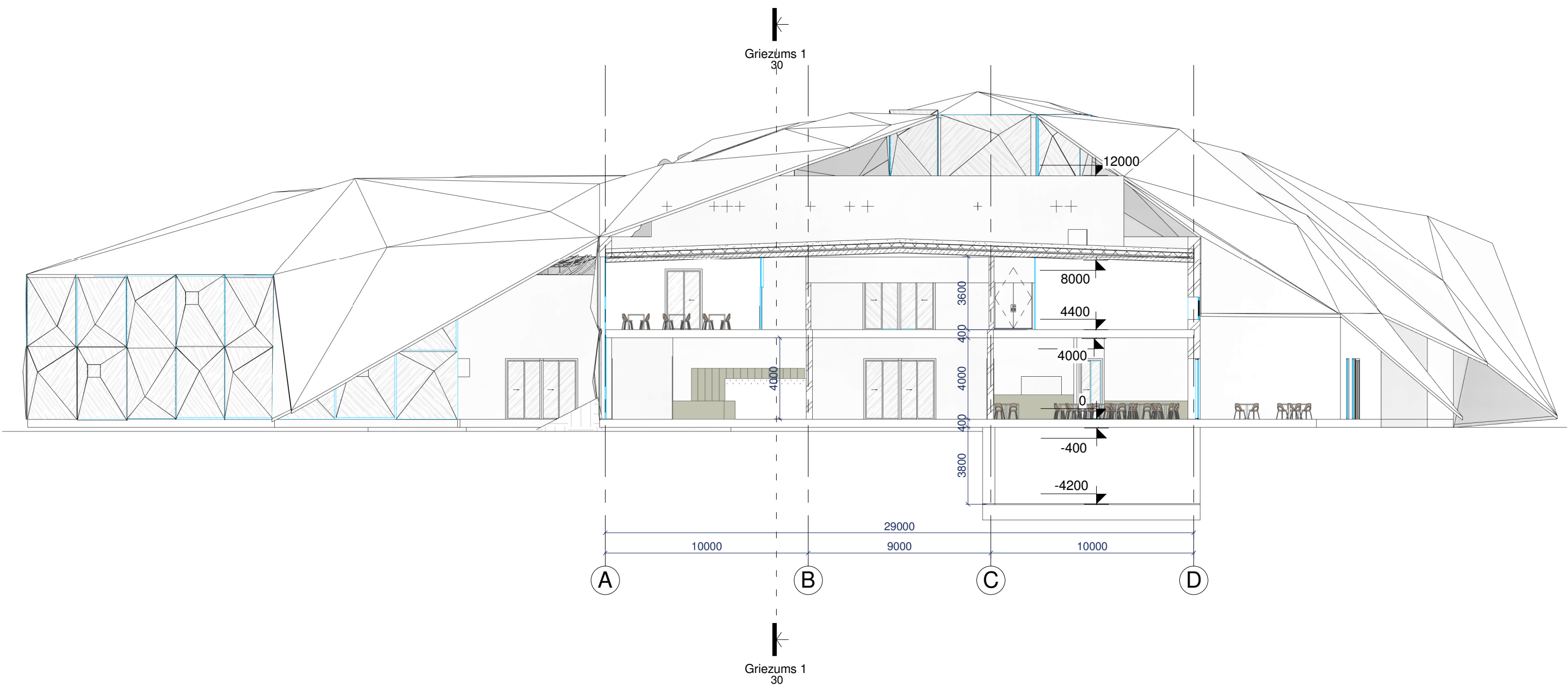
Griezums 3
